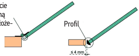
Rysunek 2 - Zabezpieczenie mechaniczne
